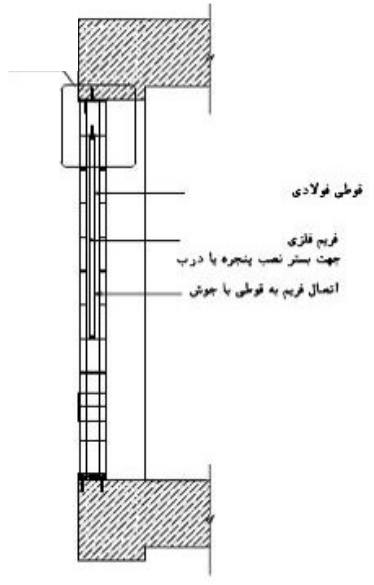
برش A-A
