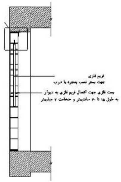
برش A-A
