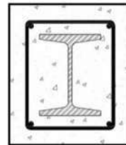
(الف) عضو محوری مختلط محاط در بتن
