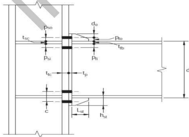
ت) هندسه اتصال فلنجی چهار پیچی با استفاده از ورق لچکی
