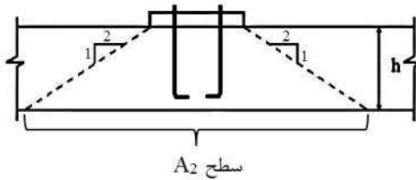
شکل ۲-۱۰-۹-۲۲: سطح اتکا در تماس با تکیه‌گاه بتنی
