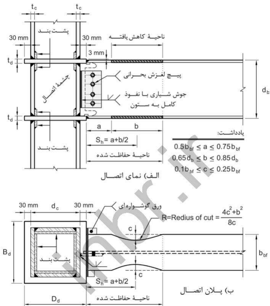
شکل ۱۰-۳-۷-۱۲: اتصال گیردار تیر با مقطع کاهش یافته و دیافراگم عبوری از ستون در قاب‌های خمشی
