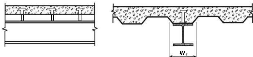
شکل ۱۰-۲-۹-۸: عرشه فولادی که کنگره‌های آن موازی با محور طولی تیر است
