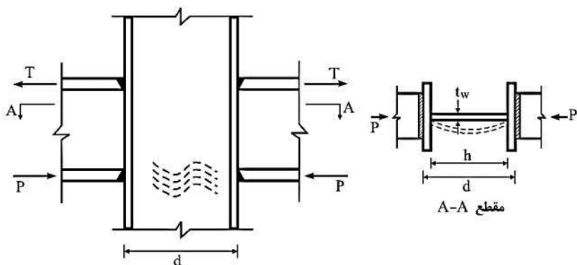
شکل ۱۰-۲-۹: ۲۷-۹-۲-۱۰. کمناش فشاری جان در مقابل یک جفت نیروی متمرکز فشاری
