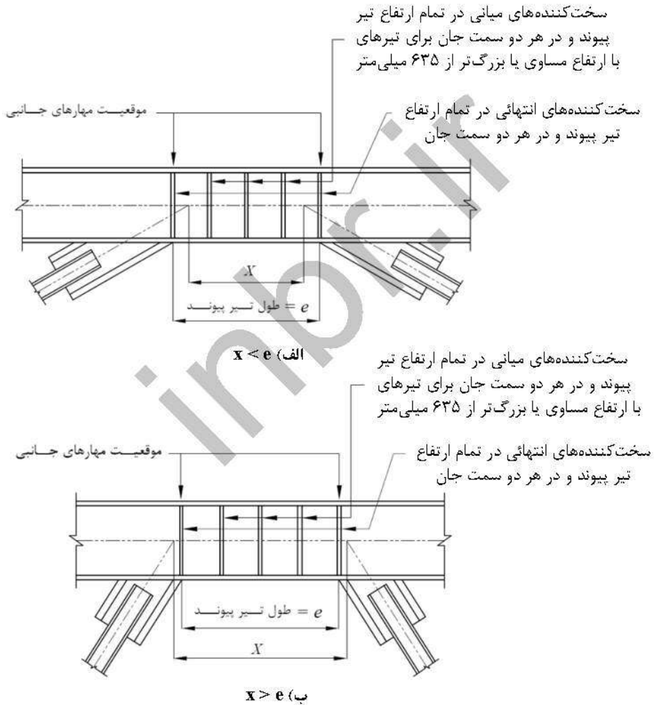
شکل ۳-۱۰-۳-۴-۳-۲: تیر پیوند با مقطع I شکل و سخت‌کننده‌های موردنیاز
