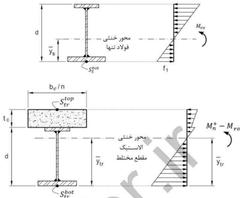
شکل ۱۰-۲-۸: توزیع الاستیک تنش در مقطع مختلط تبدیل یافته در صورت عدم استفاده از پایه‌های موقت
