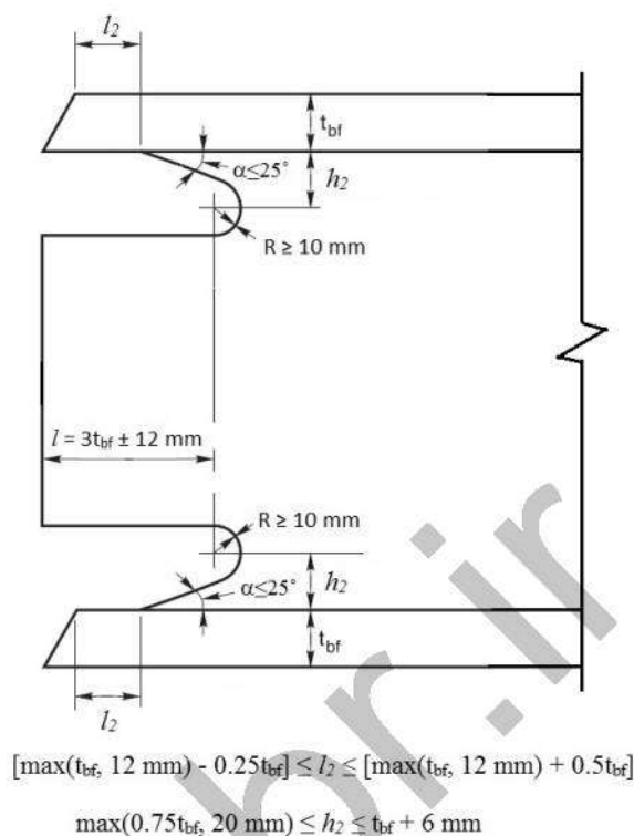
شکل ۱۰-۳-۲-۱: دیتیل جایگزین برای سوراخ‌های دسترسی اتصالات خمشی
