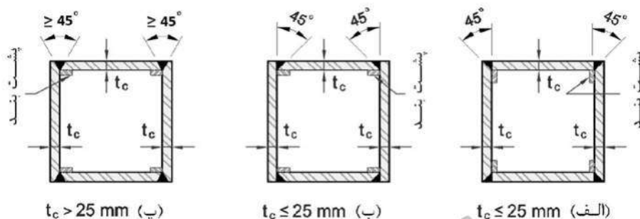
شکل ۱-۷-۳-۱۰: نحوه ساخت ستون‌های جعبه‌ای ساخته شده از ورق
