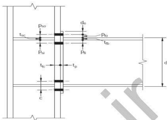
ت) هندسه اتصال فلنجی چهار پیچی بدون استفاده از ورق لچکی
