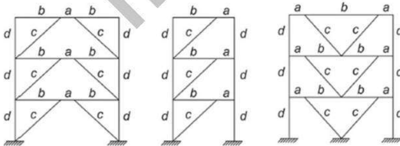
a = تیر پیوند و b = تیر خارج از ناحیه تیر پیوند c = عضو مهاربندی و d = ستون
