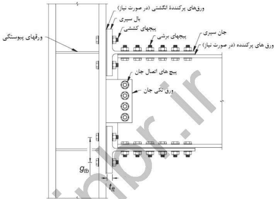
شکل ۳-۱۰-۷-۸: اتصال گیردار پیچی با جفت سپری (DT)
