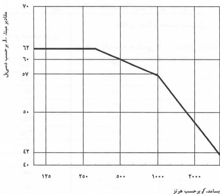
شکل ۱۸-۱-۳-۱: نمودار مقادیر مینا برای صدای کوبه‌ای، در بندهای یک‌سوم هنگامی
