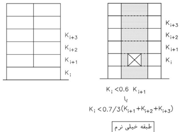
ث - نامنظمی سختی جانبی
