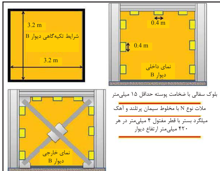
شکل پ.۲-۵- طراحی دیوار B به همراه جزئیات آن
