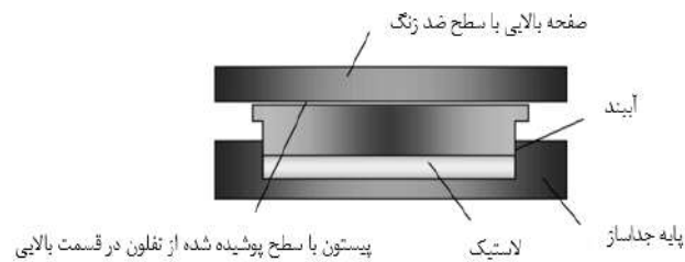
شکل ۲-۹ - جداساز کاسه‌ای
