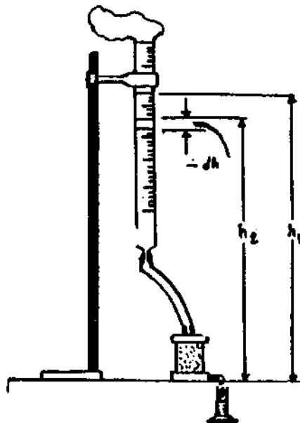
شکل ۴- دستگاه اندازه گیری تراوایی با بار افتان
