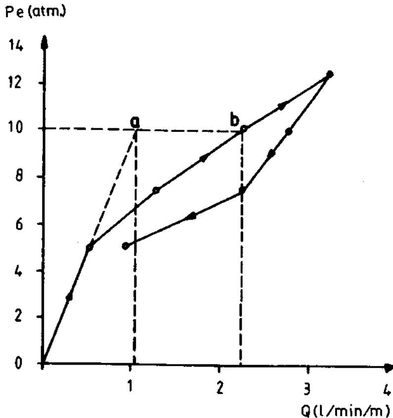
شکل ۱۰- نحوه محاسبه تراوایی و تزریق‌پذیری
